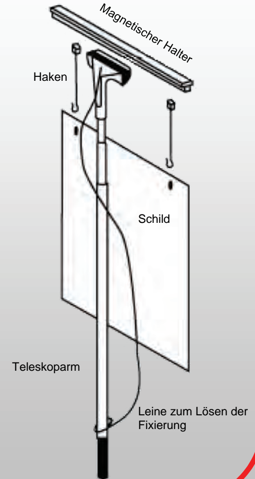
Fensterhalter mit Teleskop Montage.
